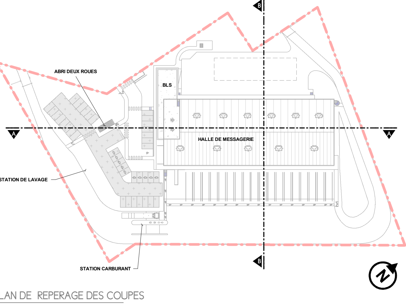
PLAN DE REPERAGE DES COUPES
